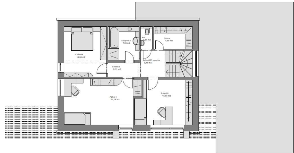
půdorys 2.NP
